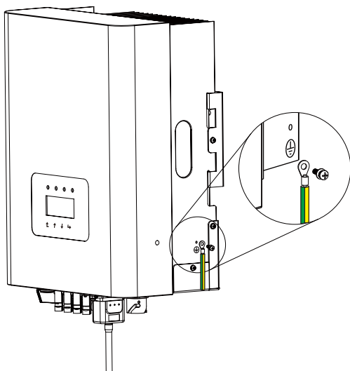
Figura 5.11 A instalação do Aterramento da Carcaça
