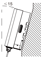
Figura 4.2 Ângulo de Instalação
