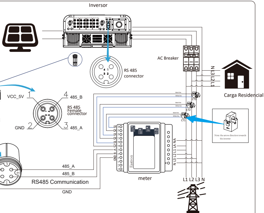
Figura 7.13 Diagrama de conexão com o medidor Eastron
