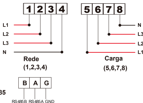
Figura 7.10 Medidor Eastron
