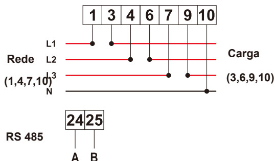
Figura 7.14 Medidor CHINT
