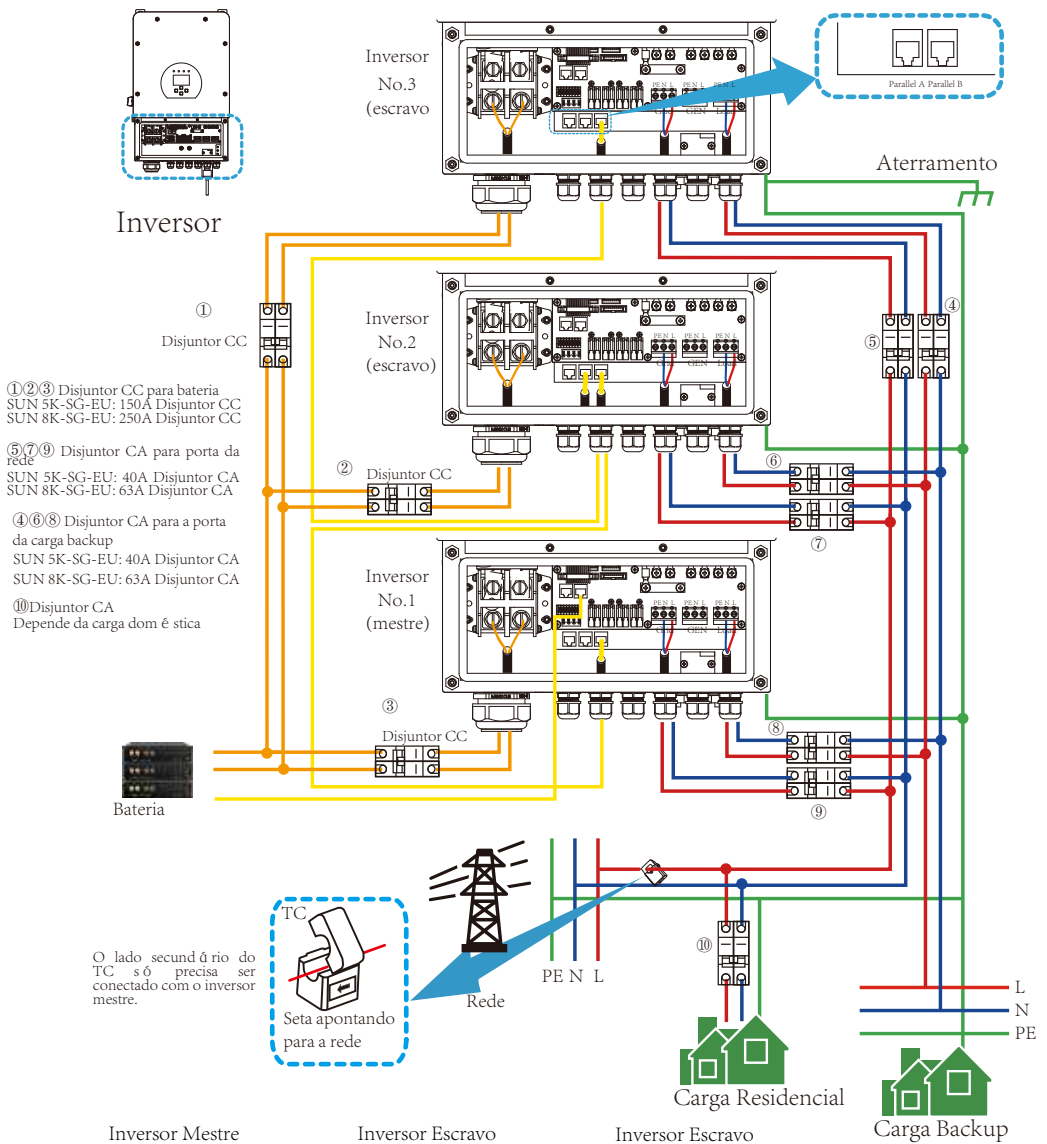
Inversor Mestre
