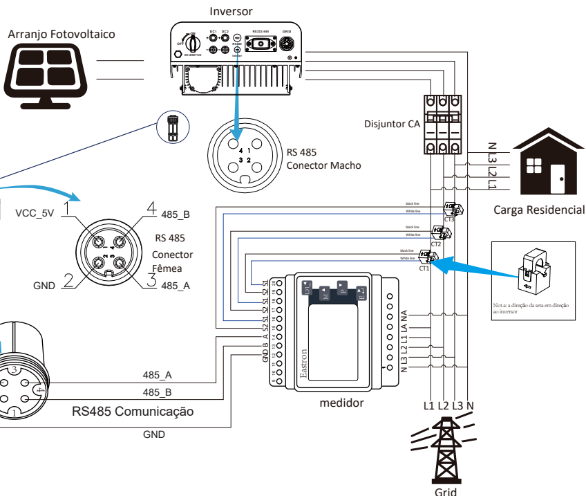
Figura 14 Diagrama da Comunicação do medidor Eastron
