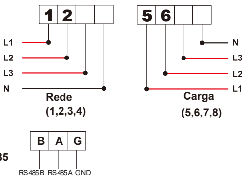
Figura 7.11 Medidor Eastron
