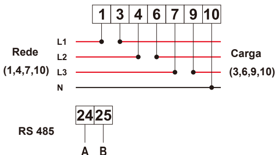
Figura 7.14 Medidor CHINT
