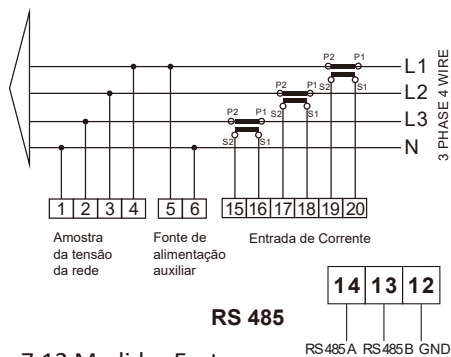
Figura 7.12 Medidor Eastron
