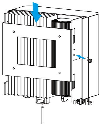
Figura 4.6 Instalação do Inversor
