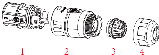
1. Soquete de Encaixe 2. Luva 3. Núcleo de Selamento 4. Porca de Selamento
