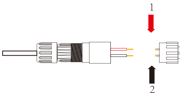
Figura 7.5 Terminal à prova d'água
