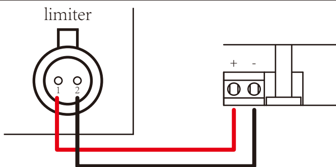
Figura 7.6 Conecte do limitador ao inversor
