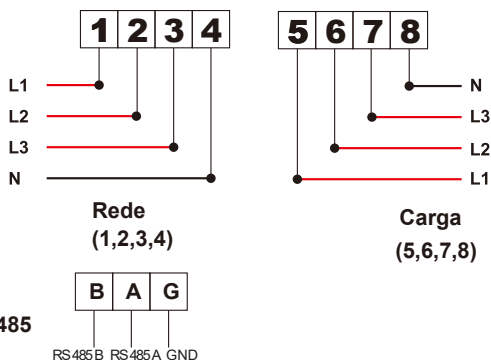
Figura 7.10 Medidor Eastron
