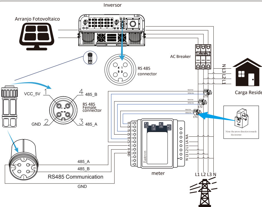
Figura 7.13 Diagrama de conexão para o medidor Eastron
