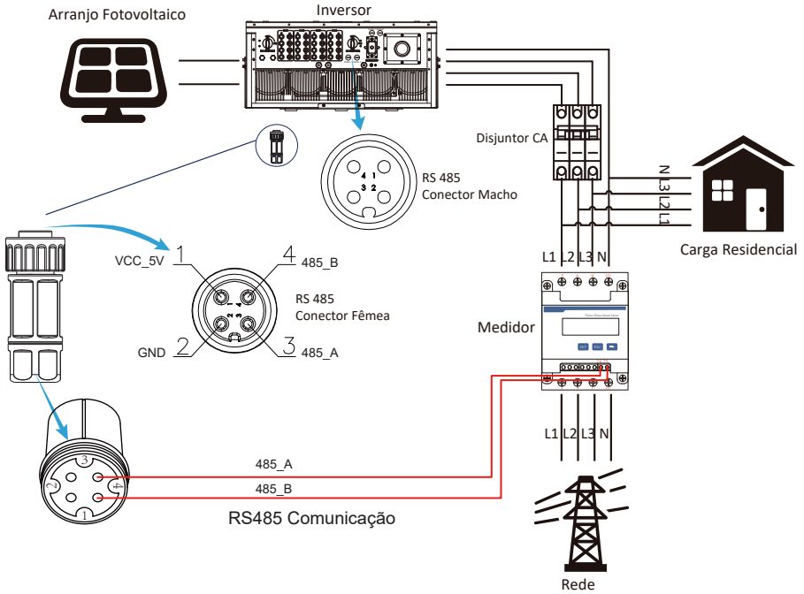
Figura 7.15 Conexão do diagrama do medidor CHINT
