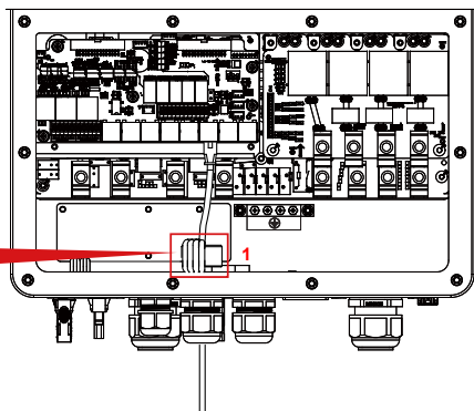
Figura 3.6 Conexão de entrada CC
