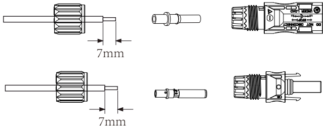
Figura 3.3 Desmontagem da porca de capa do conector
