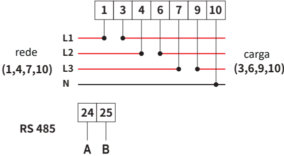
Figura 7.28 Medidor CHINT
