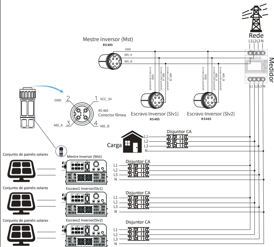
Figura 7.19 Diagrama de conexão Easton (A tabela de passagem)
