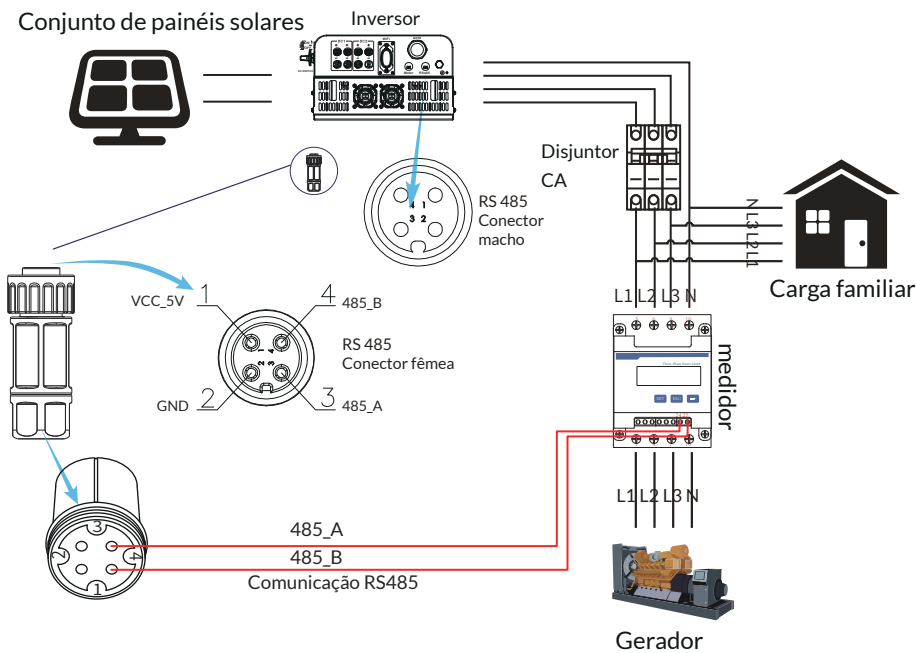
Figura 7.12 Diagrama de conexão do medidor CHINT
