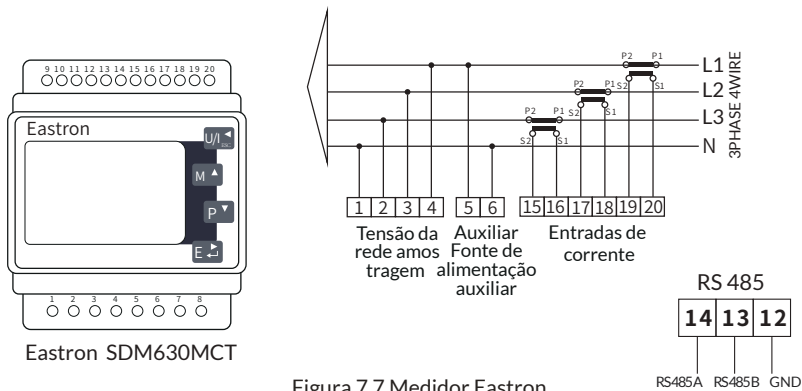
Figura 7.7 Medidor Eastron
