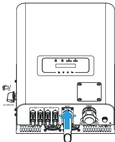
Figura 5.10 Diagrama de instalação do Datalogger
