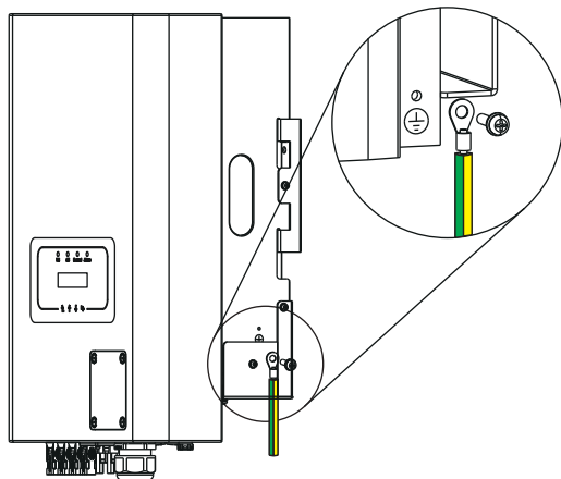
Figura 5.8 A instalação do condutor terra na carcaca
