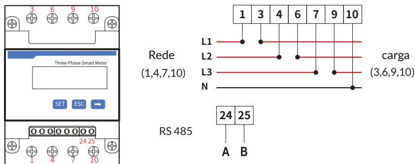
CHINT DTSU666 5(80)A
