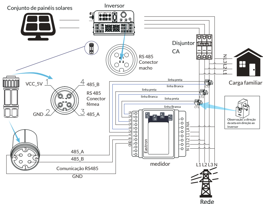
Figura 7.6 Diagrama de conexão do medidor Eastron
