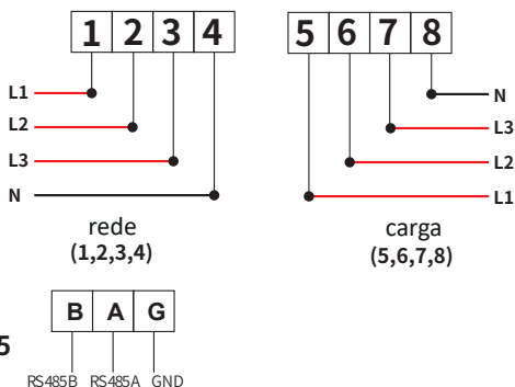
Figura 7.18 Medidor Eastron
