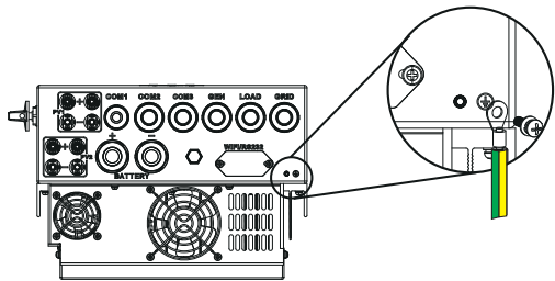
Conexão de aterramento (fios de cobre)
