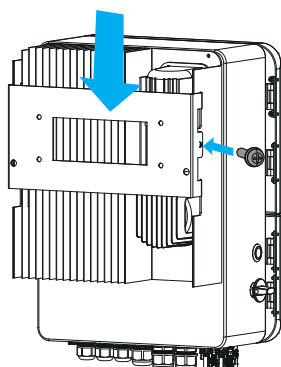
Instalação da placa suspensa do inversor
