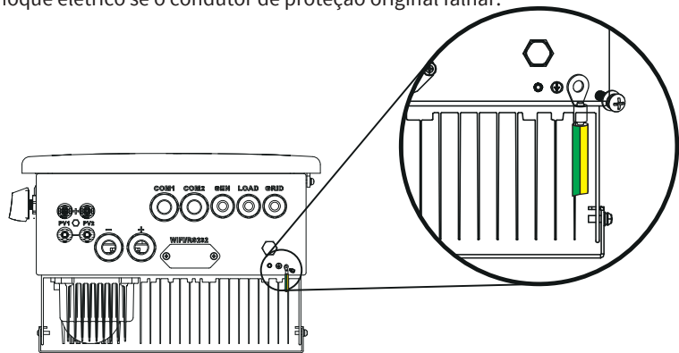
Conexão de aterramento (fios de cobre)
