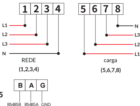
Figura 7.1 Medidor Eastron
