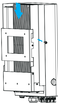
Figura 4.6 Instalação do inversor
