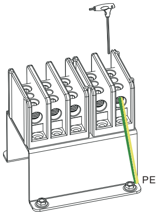
Figura 5.8 A instalação do condutor terra na carcaca
