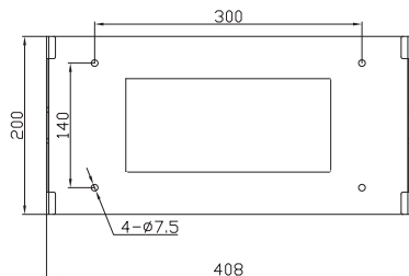
Figura 4.5 Instalação da placa de suspensão do inversor
