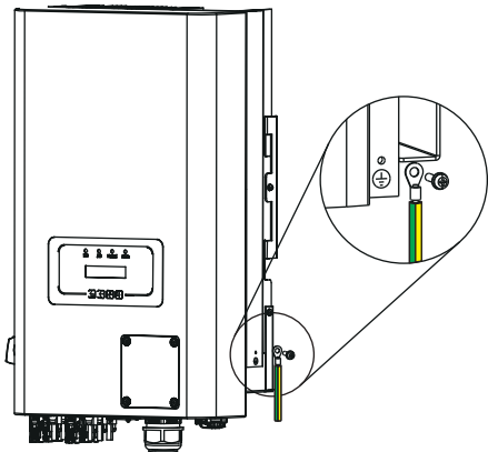
Figura 5.8 A instalação do condutor terra na carcaca
