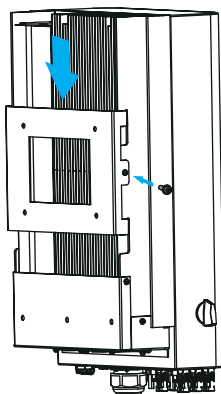
Figura 4.6 Instalação do inversor
