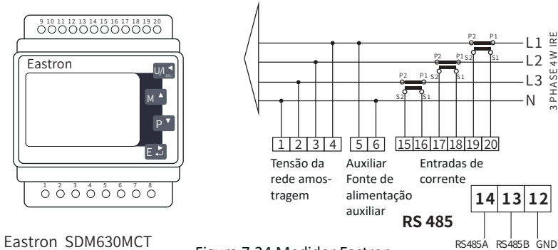
Figura 7.24 Medidor Eastron
