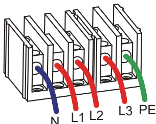
Figura 5.9 Condutor CA conectado ao terminal
