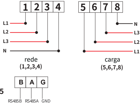
Figura 7.20 Medidor Eastron
