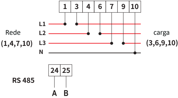
Figura 7.9 Medidor CHINT
