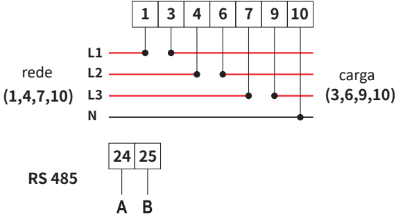
Figura 7.28 Medidor CHINT
