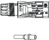
Figura 5.2 Conector CC- fêmea
