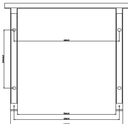
Figura 4.4 Dimensões do suporte de montagem
