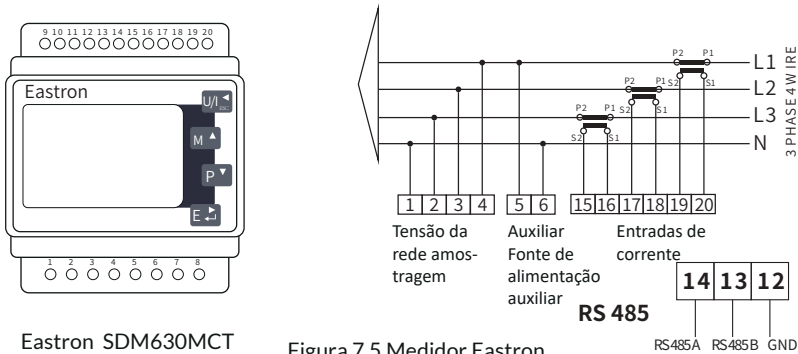
Figura 7.5 Medidor Eastron
