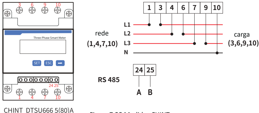
Figura 7.28 Medidor CHINT
