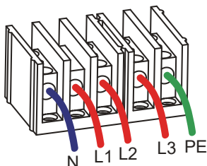
Figura 5.9 Condutor CA conectado ao terminal
