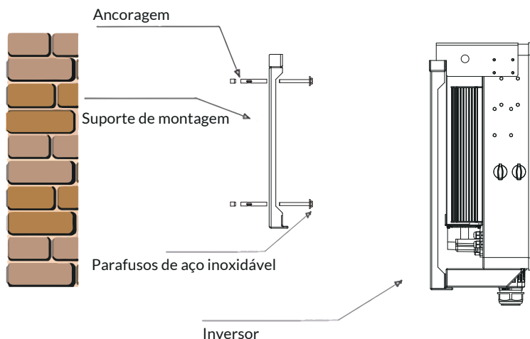
Figura 4.5 Instalação do Inversor
