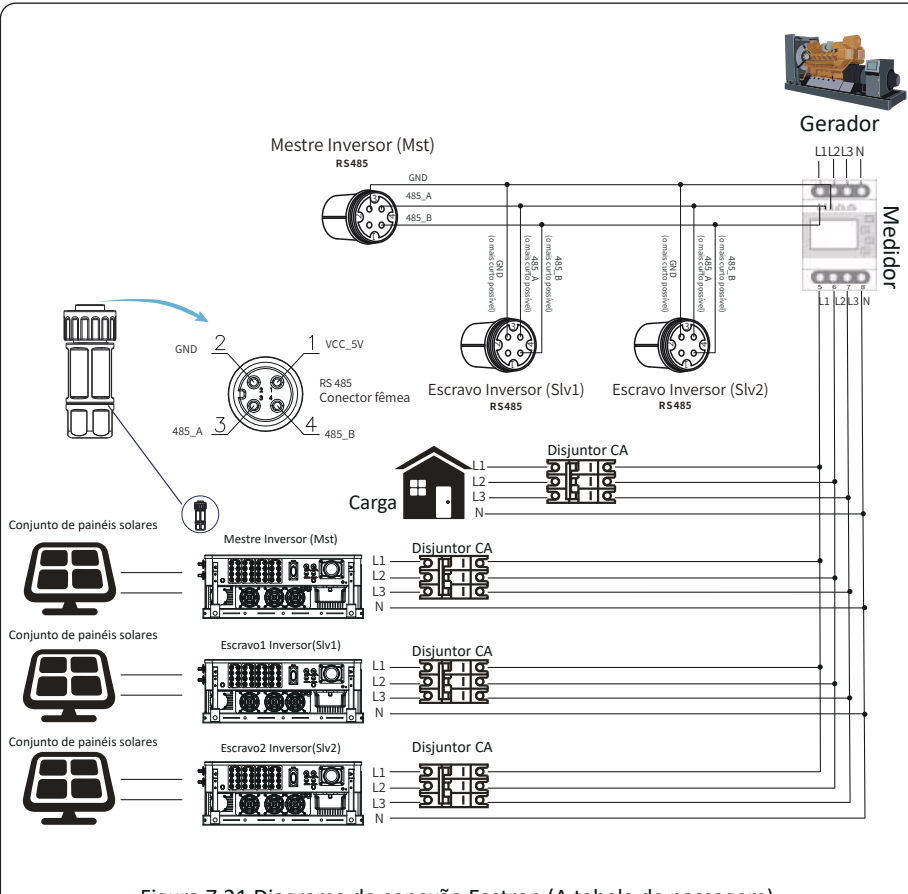
Figura 7.21 Diagrama de conexão Eastron (A tabela de passagem)
