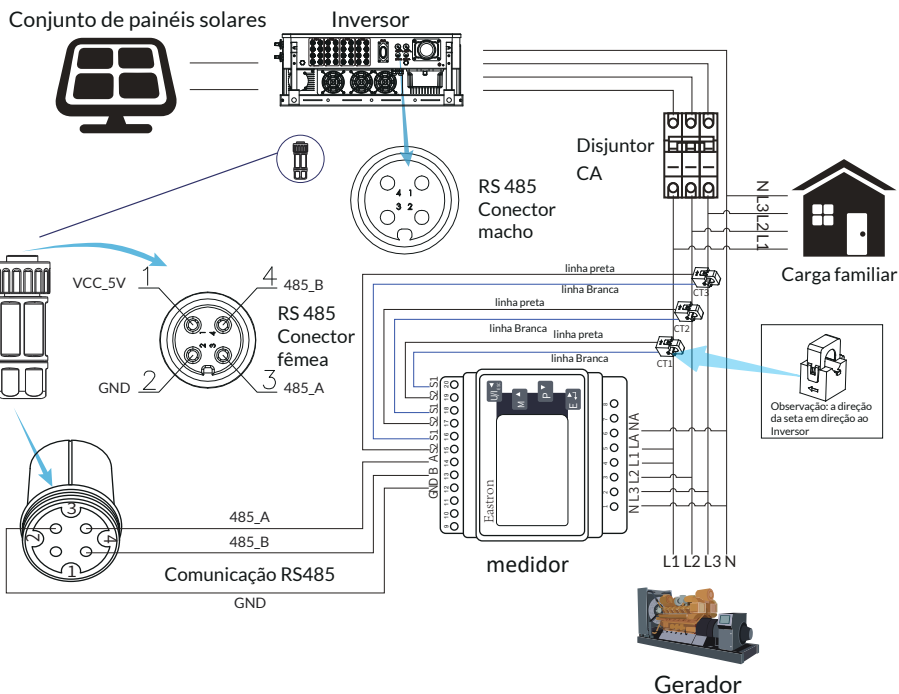
Figura 7.8 Diagrama de conexão do medidor Easton
