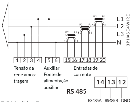
Figura 7.5 Medidor Eastron
