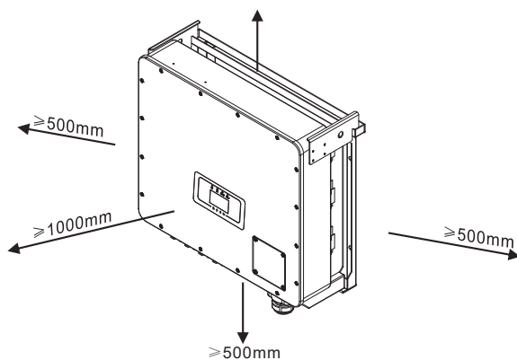
Figura 4.3 Espaço de instalação
