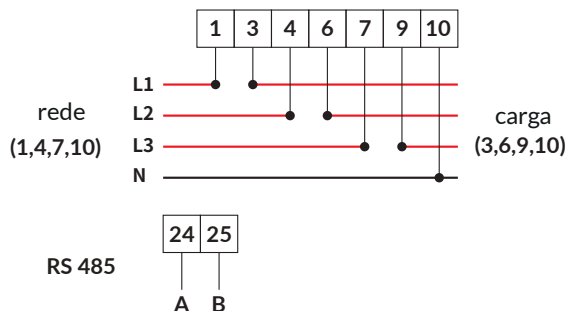
Figura 7.9 Medidor CHINT
