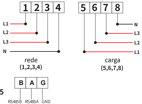
Figura 7.20 Medidor Eastron
