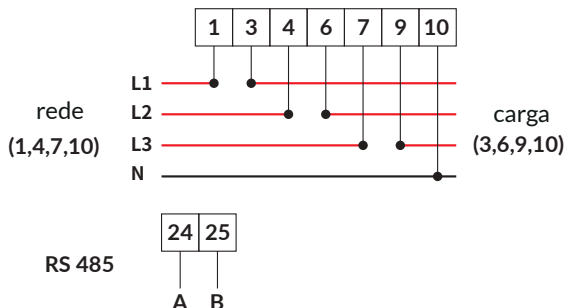
Figura 7.11 Medidor CHINT
