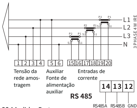
Figura 7.22 Medidor Eastron
