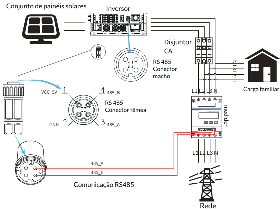
Figura 7.10 Diagrama de conexão do medidor CHINT
