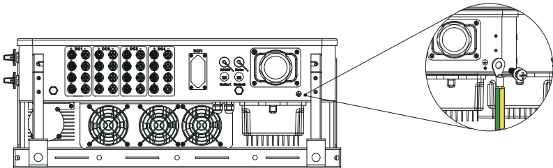
Figura 5.12 A instalação do condutor terra na carcaça
