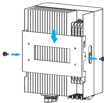
Figura 4.6 Instalação do inversor
