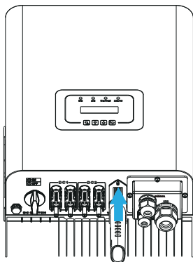
Figura 5.13 Diagrama de instalação do Datalogger
