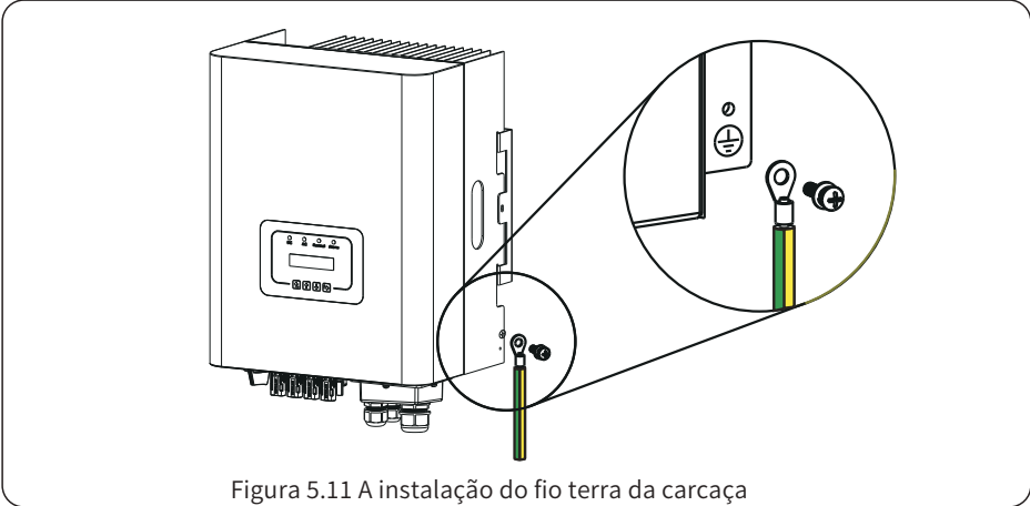
Figura 5.11 A instalação do fio terra da carcaça
