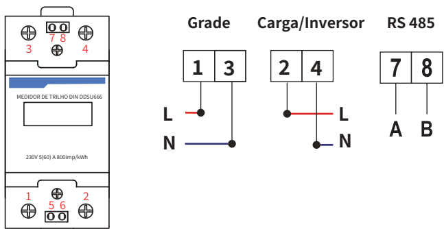
CHNT DDSU666
