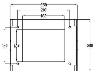
Figura 4.5 Instalação da placa de suspensão do inversor
