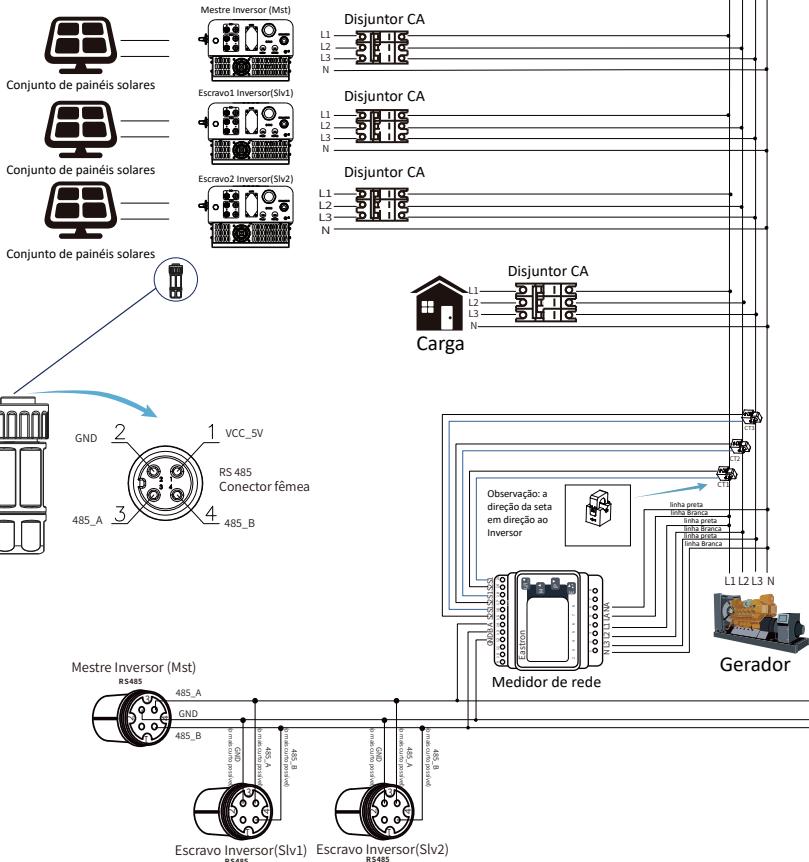
Figura 7.25 Diagrama de conexão (eletricidade Monofásica)
