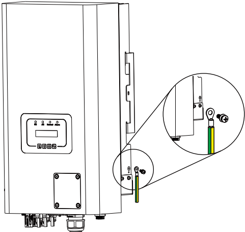
Figura 5.8 A instalação do condutor terra na carcaca
