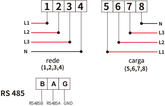
Figura 7.20 Medidor Eastron
