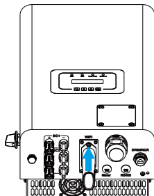
Figura 5.10 Diagrama de instalação do Datalogger
