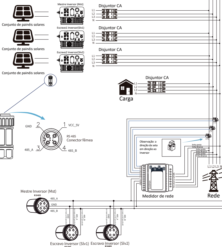
Figura 7.23 Diagrama de conexão (eletricidade Monofásica)
