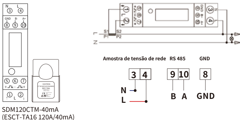
Foto 7.13 Medidor EASTRON
