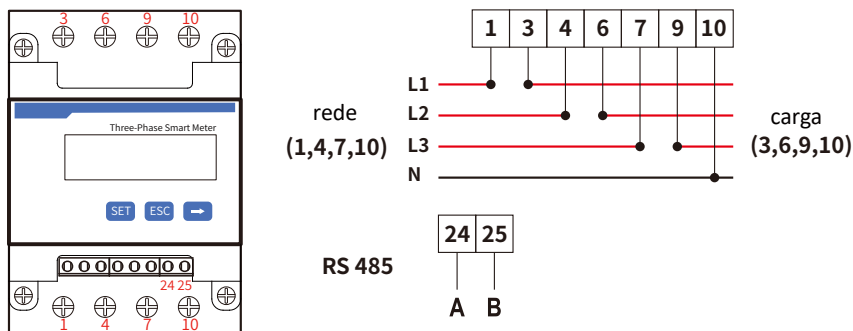
Figura 7.26 Medidor CHINT
