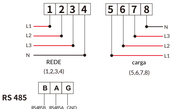
Figura 7.3 Medidor Eastron
