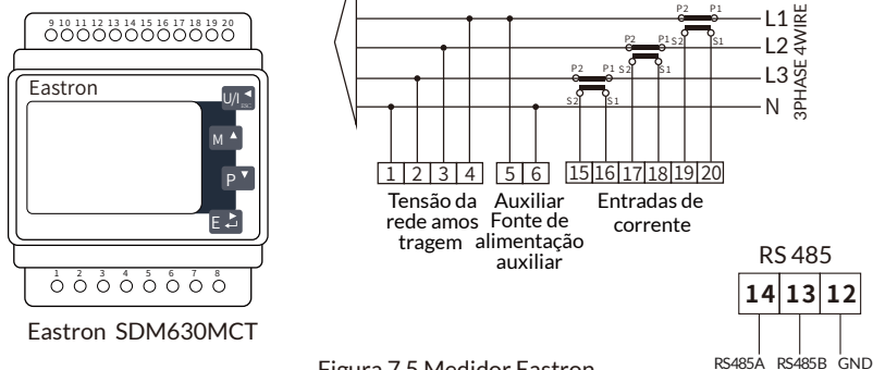
Figura 7.5 Medidor Eastron
