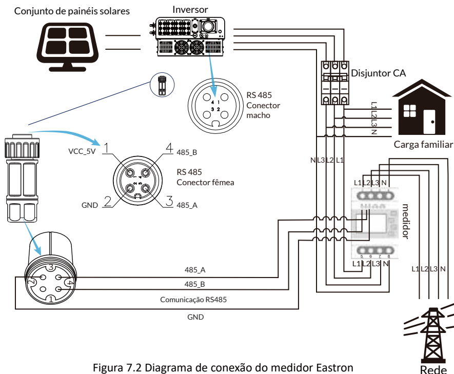
Figura 7.2 Diagrama de conexão do medidor Eastron
