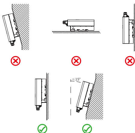
Figura 4.2 Ângulo de instalação
