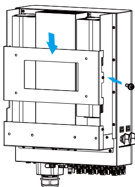
Figura 4.6 Instalação do inversor
