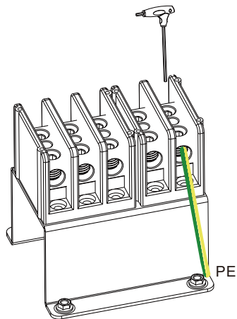
Figura 5.12 A instalação do condutor terra na carcaca
