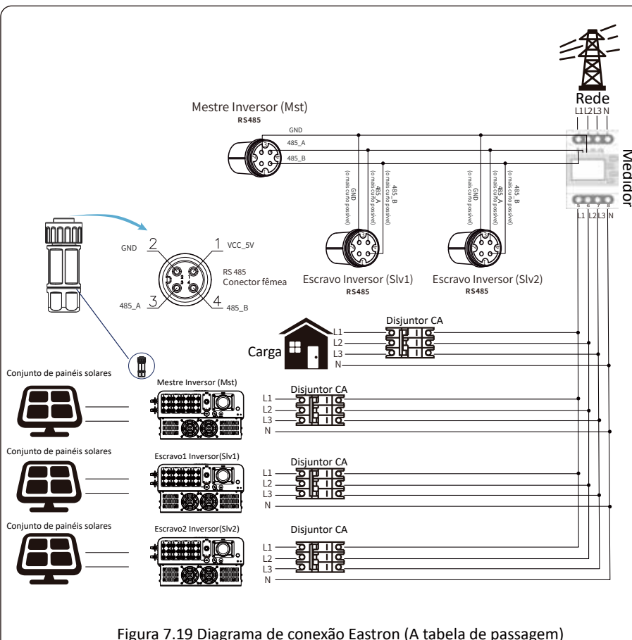
Figura 7.19 Diagrama de conexão Eastron (A tabela de passagem)
