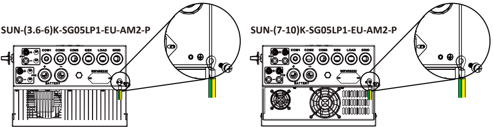
Conexão de aterramento (fios de cobre)
