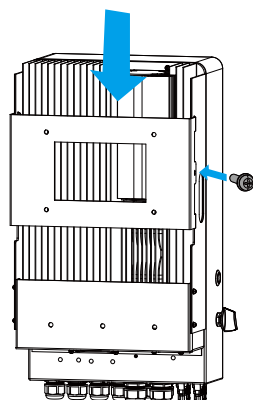
Instalação da placa suspensa do inversor
