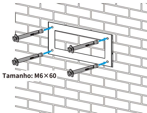
Instalação do suporte de fixação
