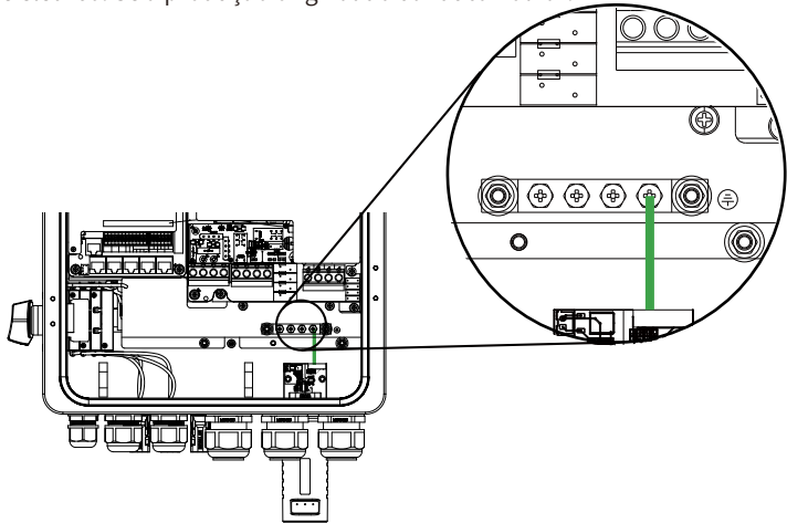
Conexão do aterramento (Condutores de cobre) (bypass)
