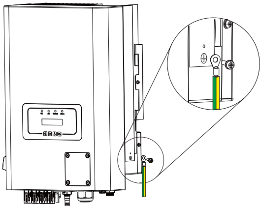
Figura 5.12 A instalação do condutor terra na carcaca
