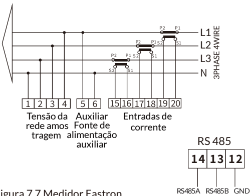
Figura 7.7 Medidor Eastron
