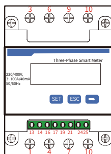
CHINT DTSU666
