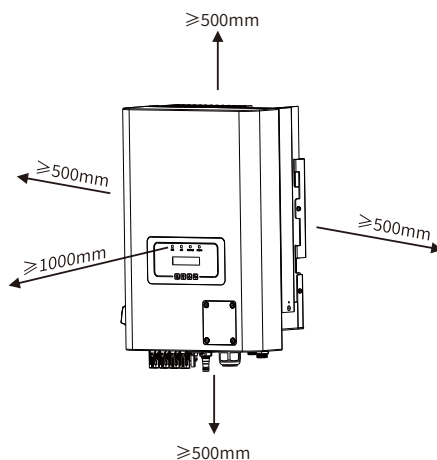
Figura 4.3 Lacuna de instalação
