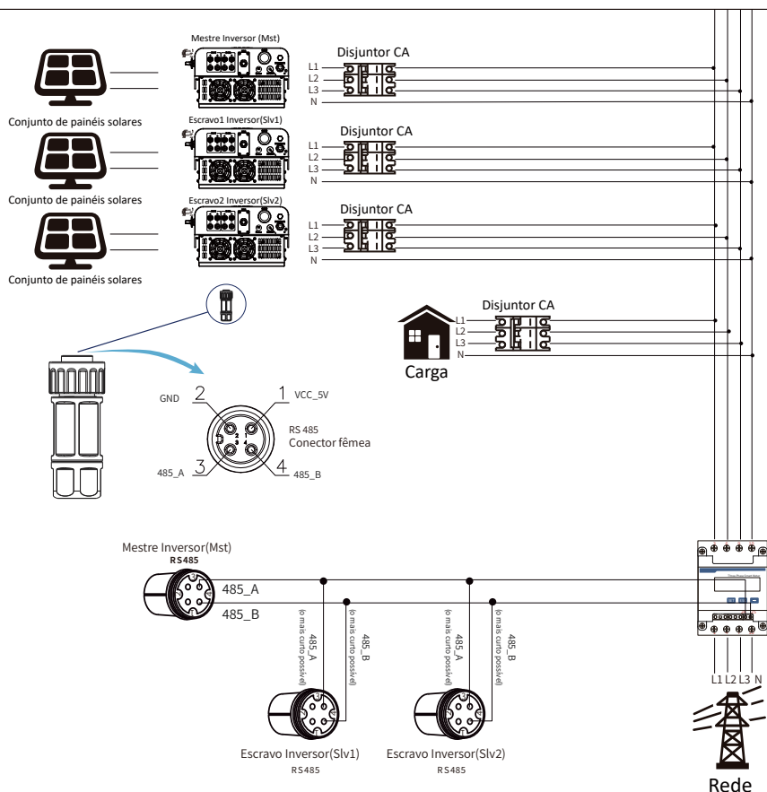
Figura 7.27 CHINT Diagrama de conexão (A tabela de passagem)
