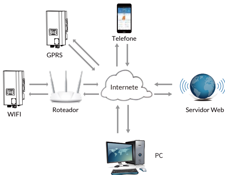
Figura 5.13 Solução de monitorização da Internet
