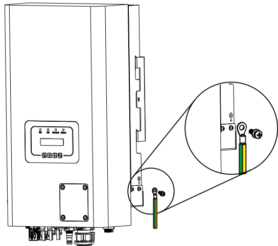
Figura 5.12 A instalação do condutor terra na carcaca
