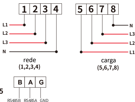
Figura 7.18 Medidor Eastron
