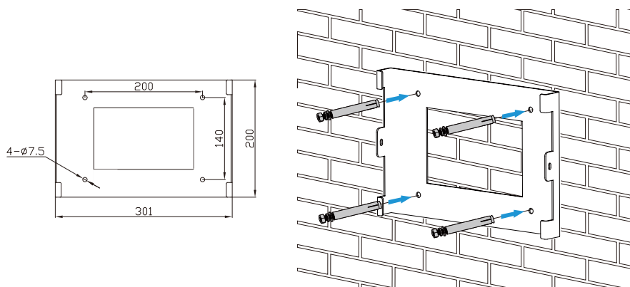
Figura 4.5 Instalação da placa de suspensão do inversor
