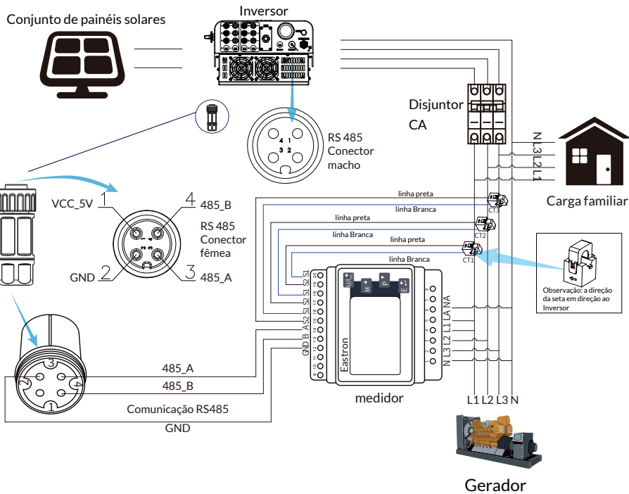
Figura 7.8 Diagrama de conexão do medidor Eastron
