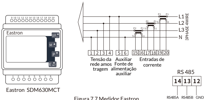
Figura 7.7 Medidor Eastron
