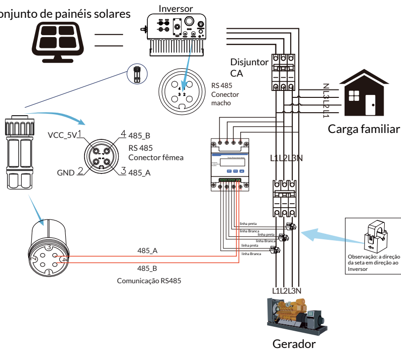
Figura 7.16 Diagrama de conexão do medidor CHINT
