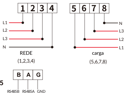
Figura 7.3 Medidor Eastron
