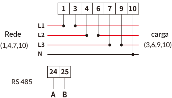
Figura 7.11 Medidor CHINT
