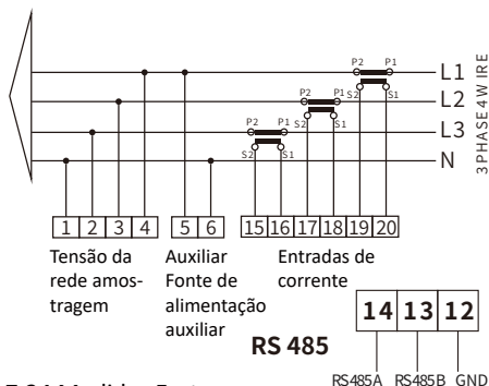
Figura 7.24 Medidor Eastron
