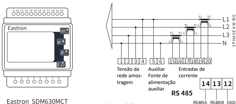
Figura 7.22 Medidor Eastron
