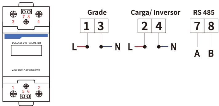
CHINT DDSU666
