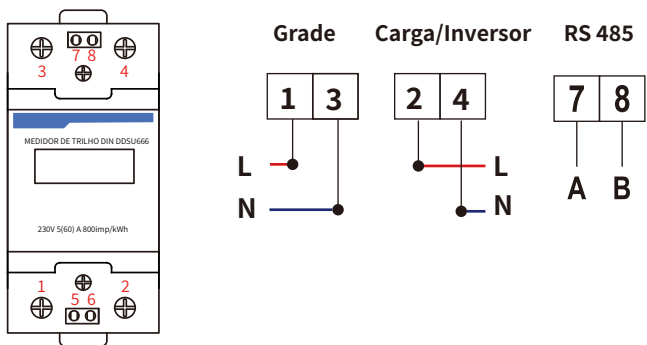
CHINT DDSU666
