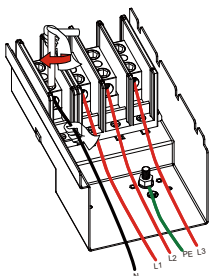
Figura 5.9 Condutor CA conectado ao terminal
