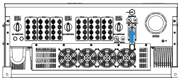
Figura 5.14 Diagrama de instalação do registador de dados
