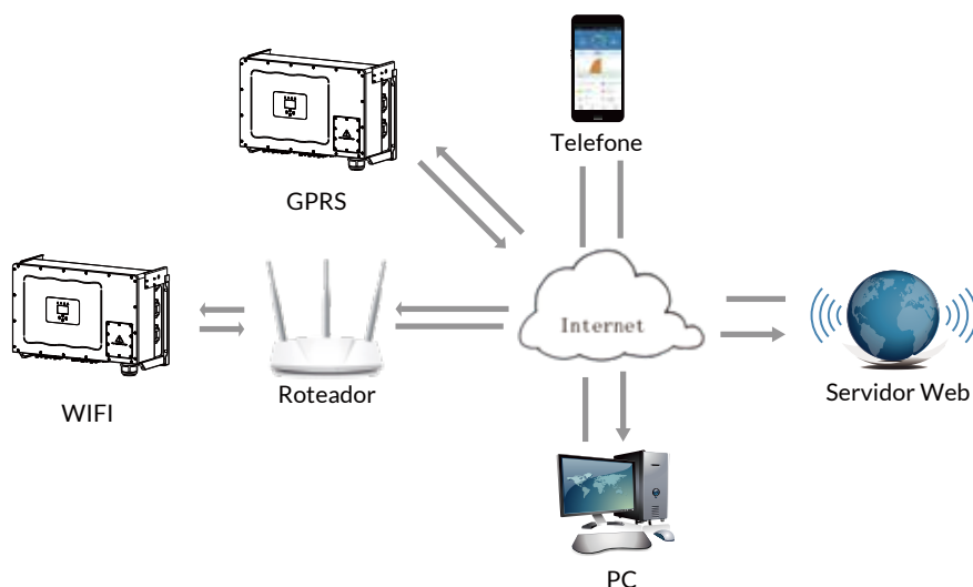
Figura 5.13 Solução de monitorização da Internet
