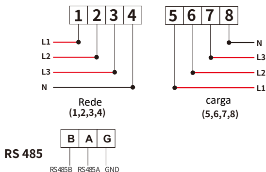
Figura 7.3 Medidor Eastron
