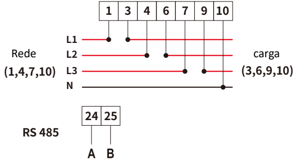
Figura 7.9 Medidor CHINT
