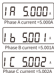
Figura 7.13 Medidor CHINT
