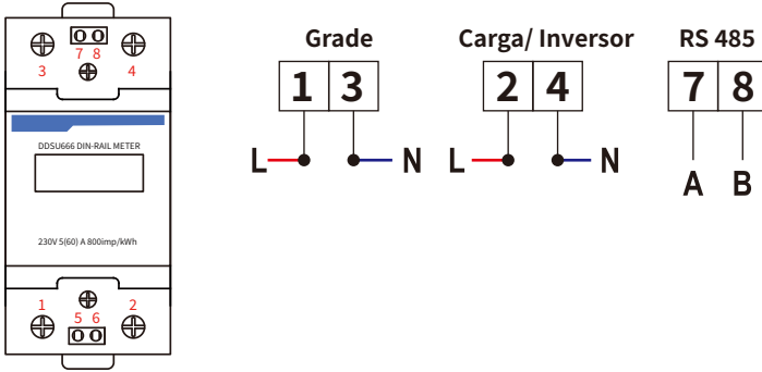
CHINT DDSU666
