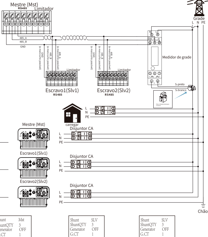
Pic 7.14 Diagrama de conexão Eastron (a tabela de passagem)
