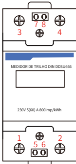
CHINT DDSU666
