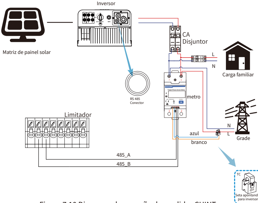
Figura 7.10 Diagrama de conexão do medidor CHINT
