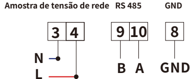
Foto 7.13 Medidor EASTRON
