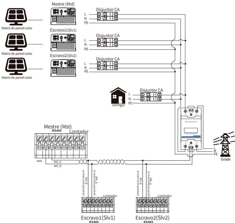
Pic 7.15 Medidor CHINT
