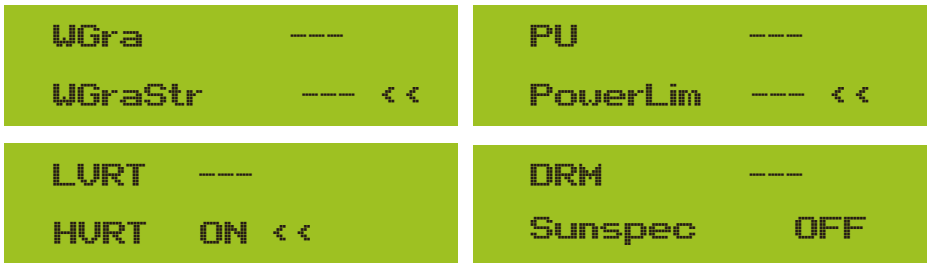
Foto 8.33 queda de potência ativa
