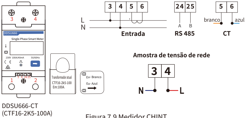
Figura 7.9 Medidor CHINT
