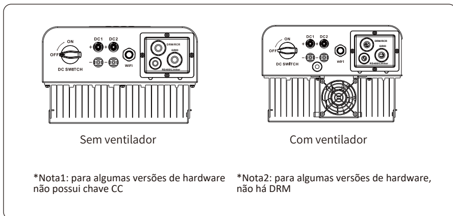
Figura 1.2 Vista inferior
