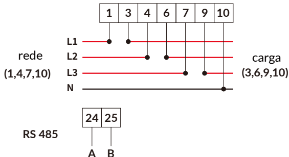
Figura 7.9 Medidor CHINT
