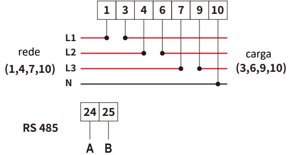
Figura 7.26 Medidor CHINT
