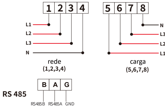
Figura 7.20 Medidor Eastron
