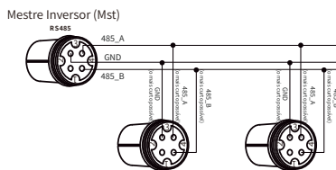
Figura 7.25 Diagrama de conexão (eletricidade Monofásica)
