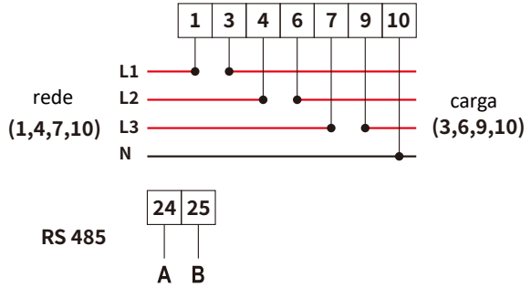
Figura 7.26 Medidor CHINT
