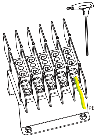
Figura 5.12 A instalação do condutor terra na carcaca
