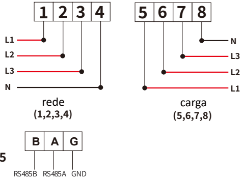
Figura 7.18 Medidor Eastron
