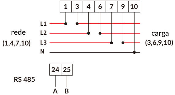
Figura 7.11 Medidor CHINT
