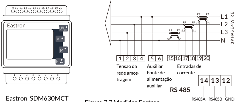
Figura 7.7 Medidor Eastron
