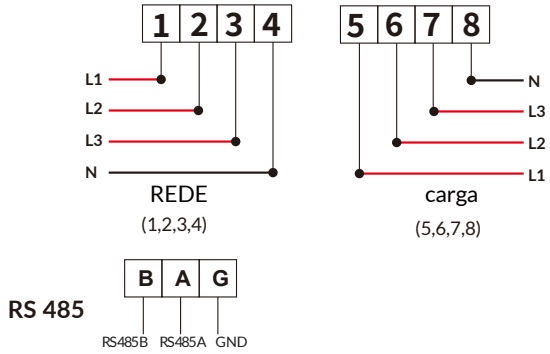
Figura 7.3 Medidor Eastron
