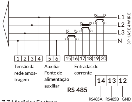
Figura 7.7 Medidor Eastron
