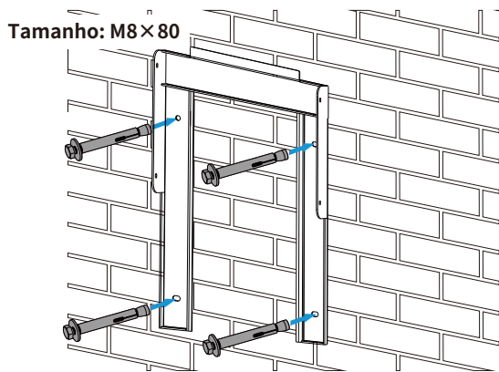
Instalação do suporte de fixação
