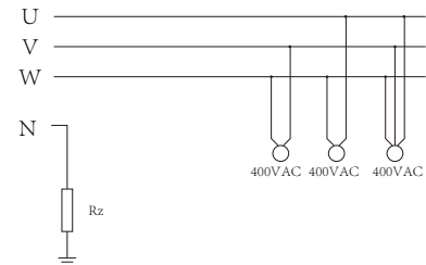
Rz: Resistência de terra de grande dimensão. Ou o sistema não tem linha neutra.
