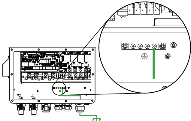
Conexão do aterramento (Condutores de cobre) (bypass)
