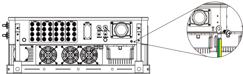
Figura 5.12 A instalação do condutor terra na carcaça
