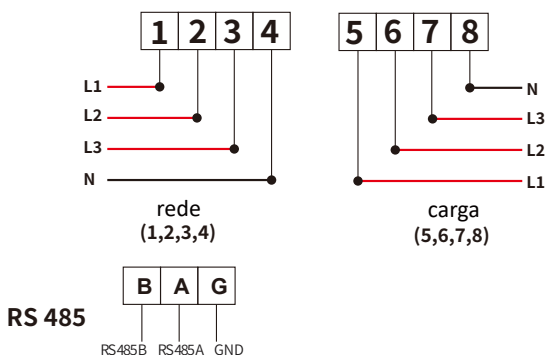
Figura 7.18 Medidor Eastron
