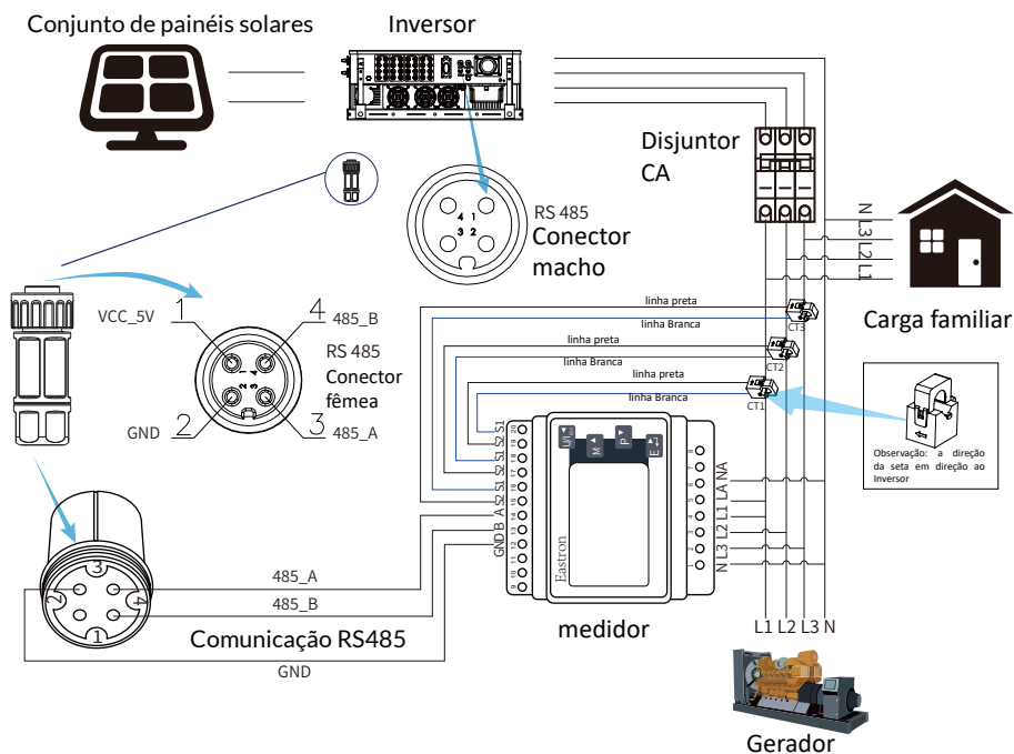
Figura 7.8 Diagrama de conexão do medidor Eastron
