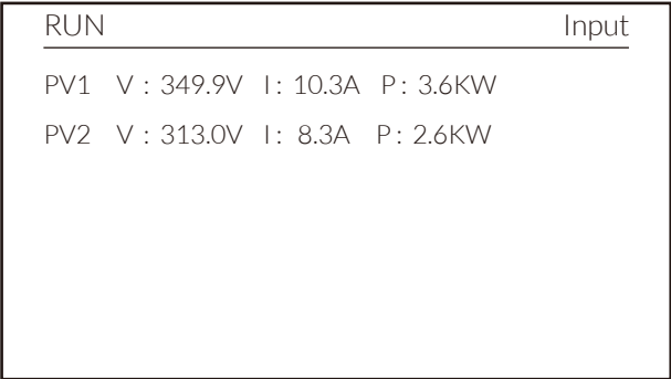
Figura 8.2 Informações sobre a entrada fotovoltaica e a corrente CC
