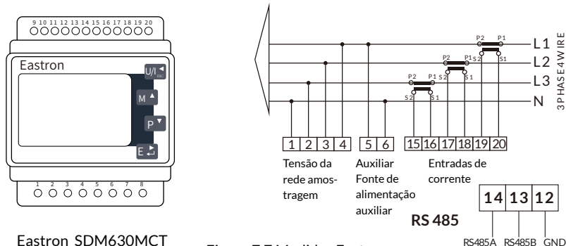
Figura 7.7 Medidor Eastron
